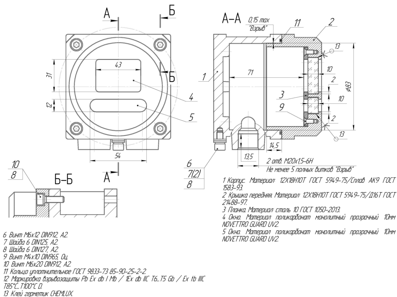
Рисунок А2 – Чертеж безопасности
