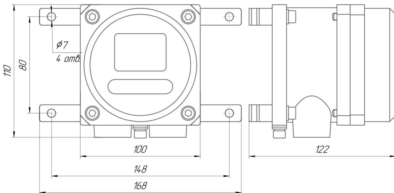
Рисунок А1 – Габаритные размеры видеокамеры АйТек ПРО А5-Exd
